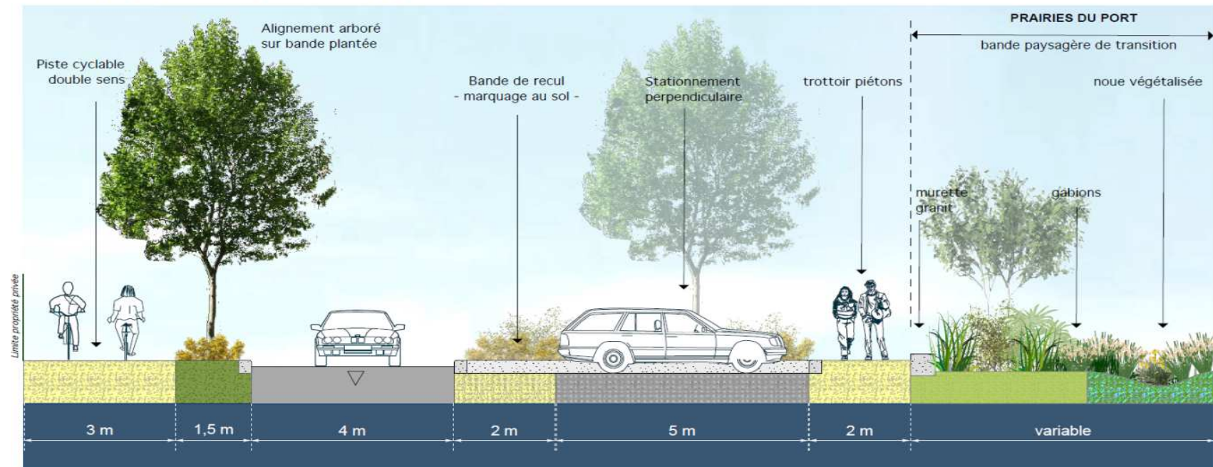
COUPE DE PRINCIPE SUR LA RUE DU PORT
